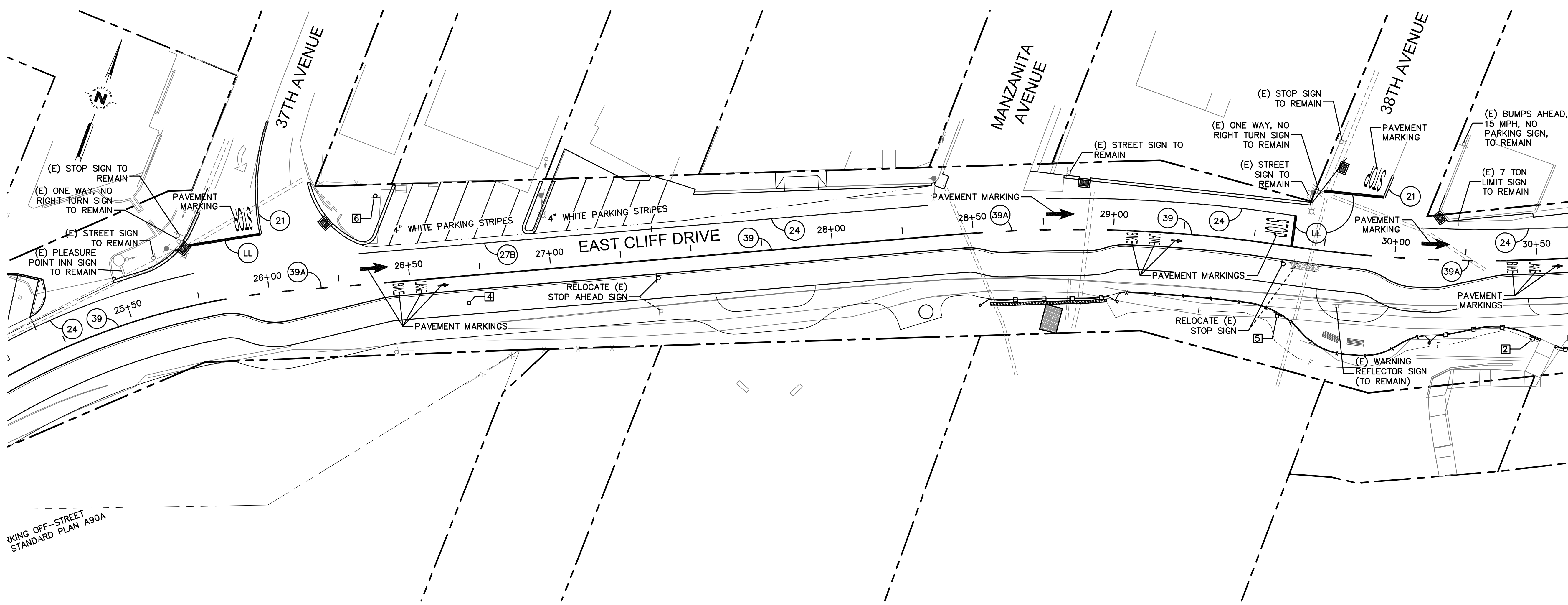
STRIPING AND SIGNAGE PLAN STA 20+00 - 30+00 SCALE: 1" = 20'
